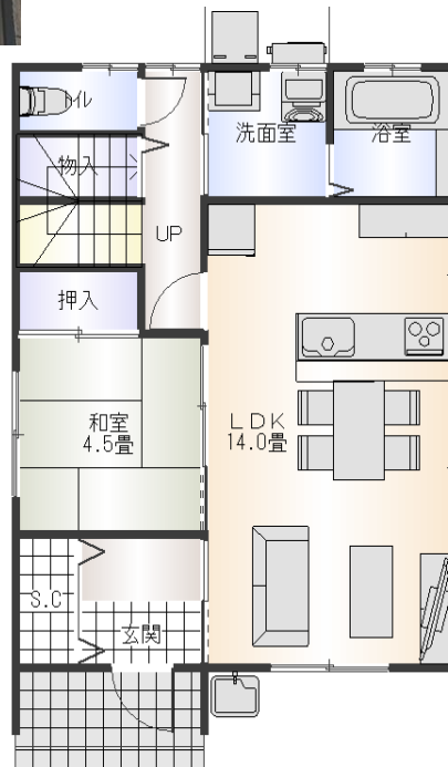
1階平面図
